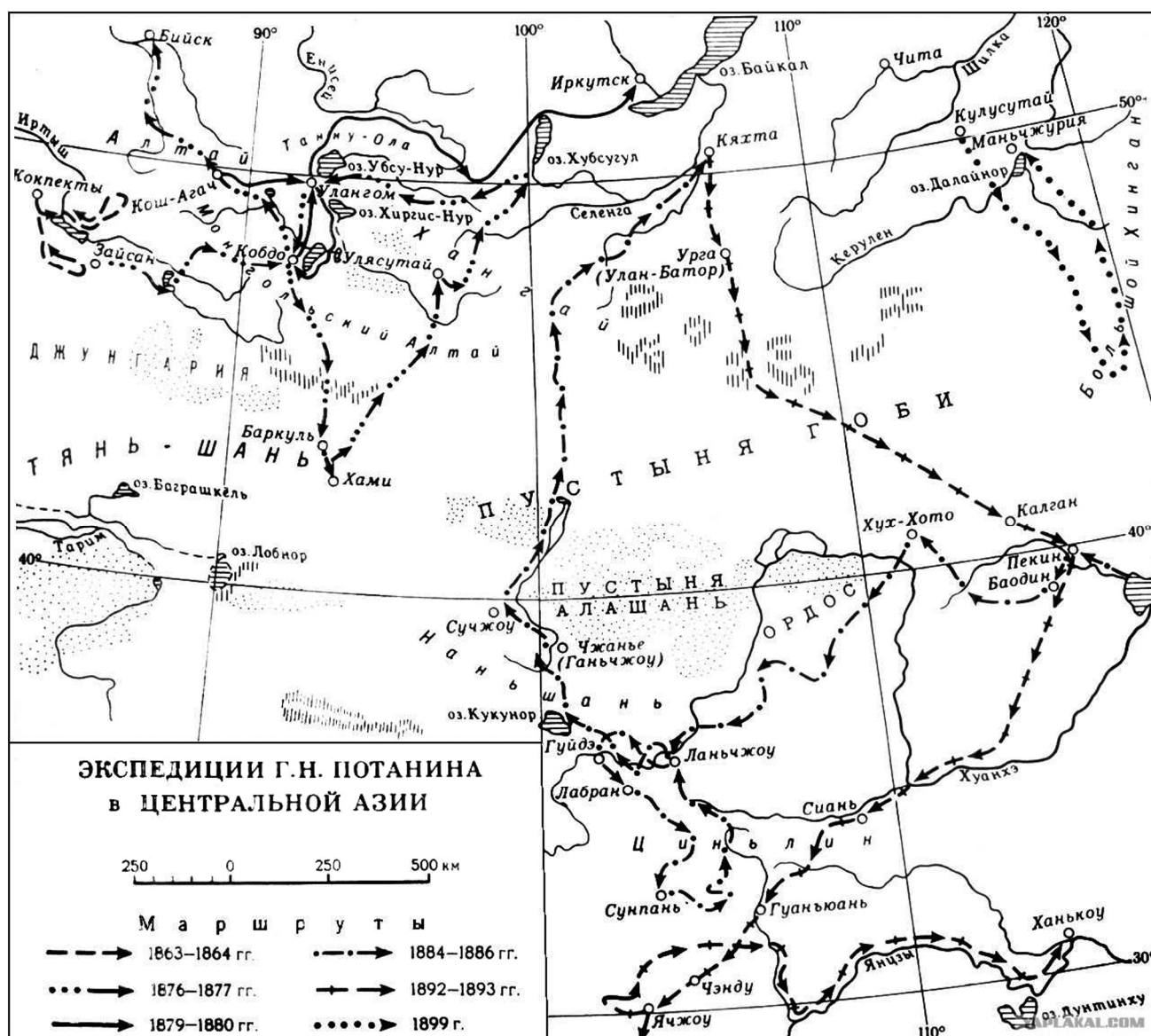
Маршруты экспедиций Г. Н. Потанина в Центральной Азии 1884—1886, 1892—1893, 1899 гг.
